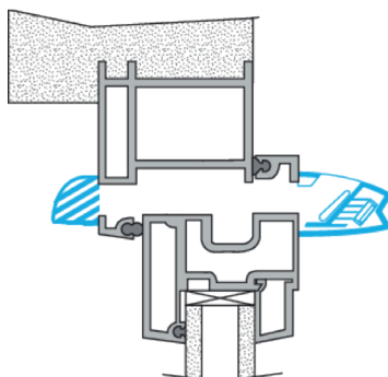
Mise en œuvre entrée d'air EHB2
