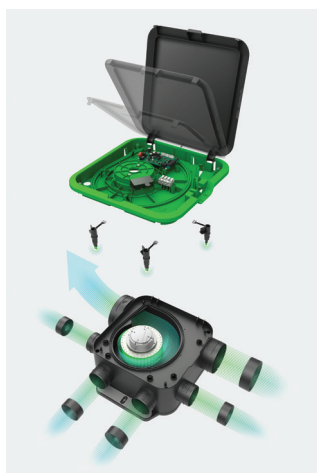
Fonctionnement en vue éclatée
