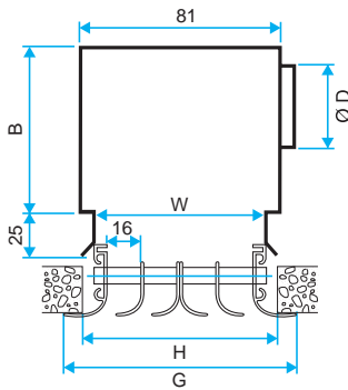
Diffuseur ALD 610 - 620
