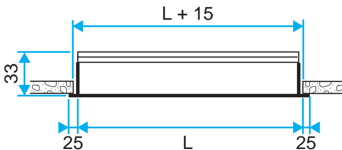
Diffuseur ALD 610 - 620
