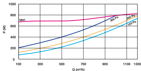
Caractéristiques aérauliques et acoustiques DFE 1200 micro-watt
