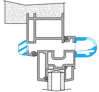
Vue en coupe entrée d'air EMMA
