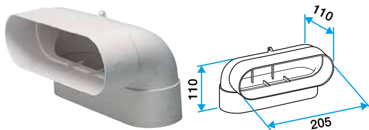
Gomito verticale a 90°
