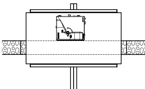
Messa in opera soletta calcestruzzo
