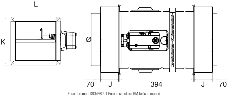
Encombrement ISONE®2.1 Europe circulaire GM télécommandé
