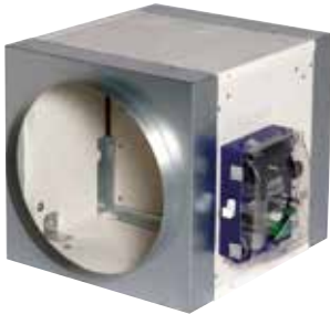
ISONO 1500 a Ghiera
