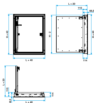
Ingombri OPTONE "Classic" 1V con controtelaio (mm)
