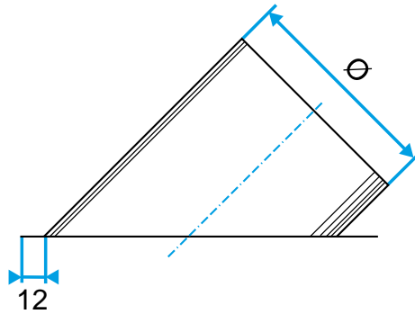
Schéma d'encombrement Piquage Oblique sur Plat 45°
