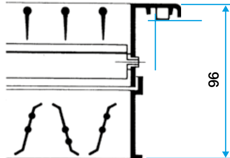
Griglia SC 102 D con serranda AGB o SGS montata
