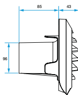
Encombrement Auvent EHT 2 -EFT 2
