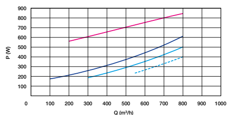
Débit et puissance VEX520
