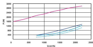
Débit et puissance VEX540
